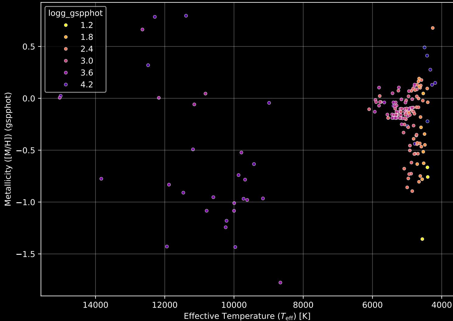
APOGEE DR17 Field: [221+04] Stellar Population Parameters (n= 172)
